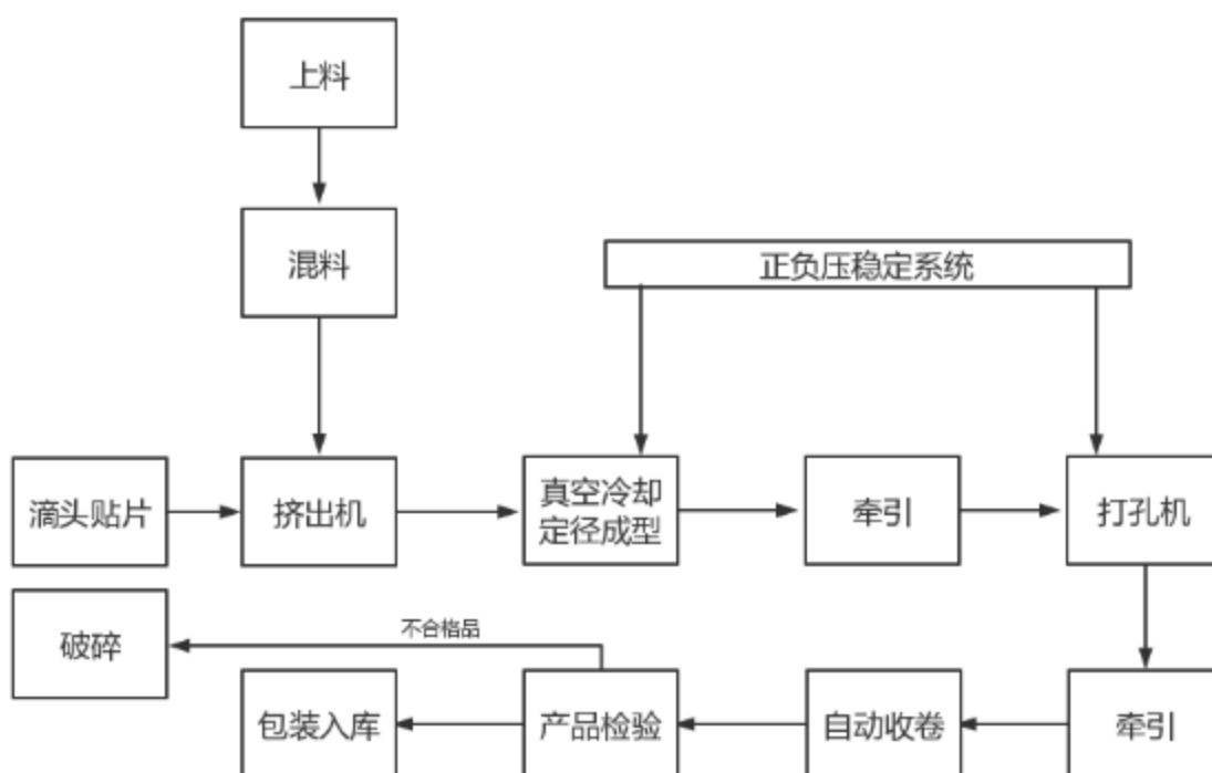
图 2.1 工艺流程图
